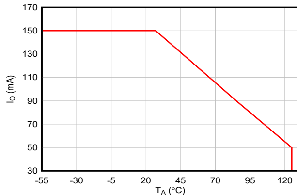
图 6-1. 典型最大负载电流与温度间的关系
