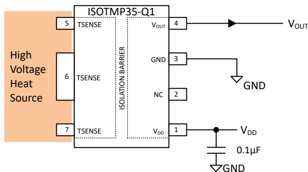
图 7-3. Typical ISOTMP35-Q1 Circuit
