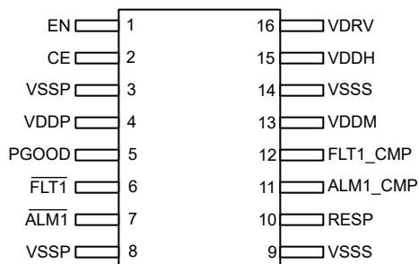
图 5-4. TPSI313x DVX 封装，16 引脚 SSOP（顶视图）
