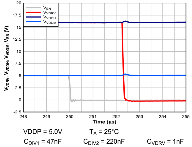
图 6-4. t_{HL\_VDRV}
