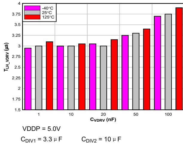
图 6-5. t_{LH\_VDRV} 与 C_{VDRV}
