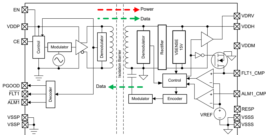
图 8-4. TPSI313x
