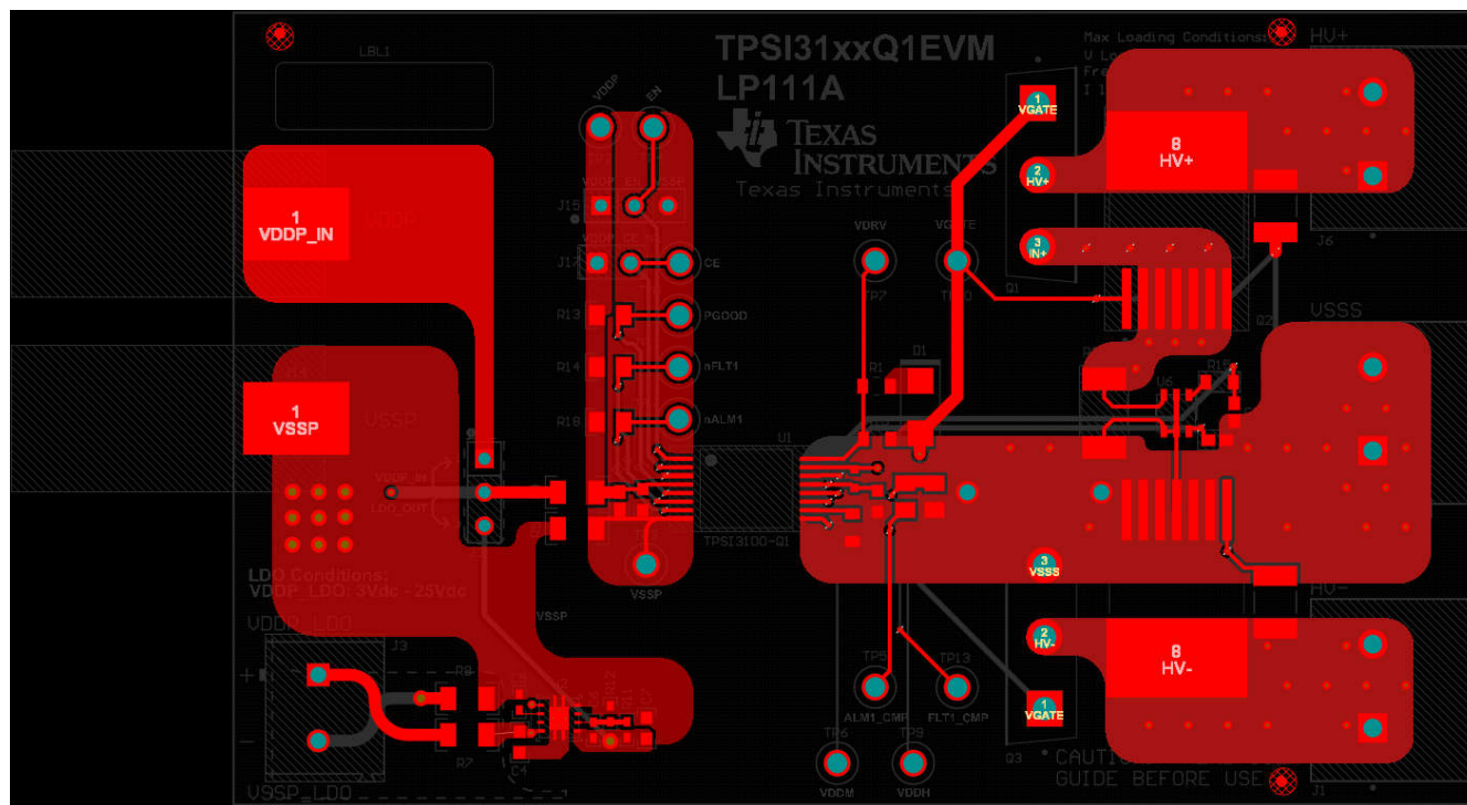
图 9-4. 顶层
