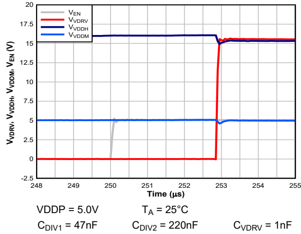
图 6-3. t_{LH\_VDRV}
