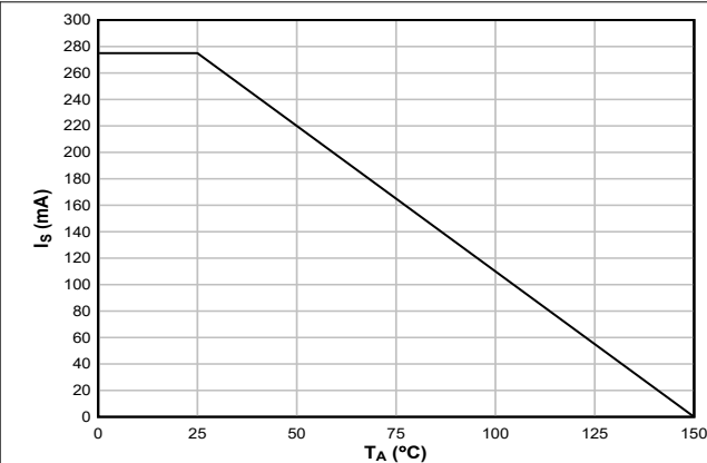
图 6-1. 根据 VDE 和 IEC 标准限制电流的热降额曲线
