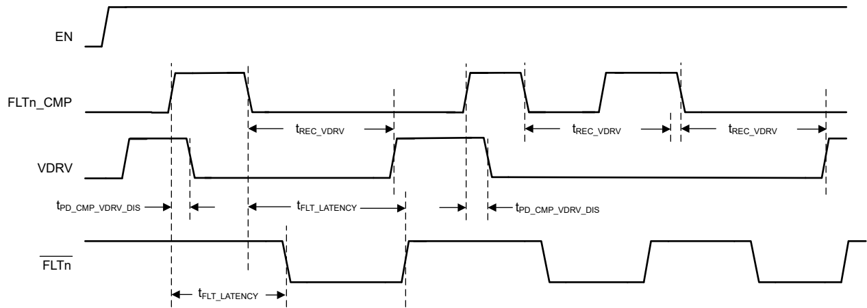
图 7-2. VDRV 自动恢复时序 ( CE = 1 或 CE = VDDP )
