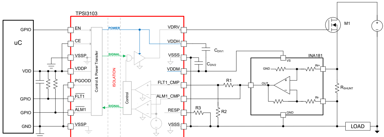
图 9-1. 典型的过流保护应用
