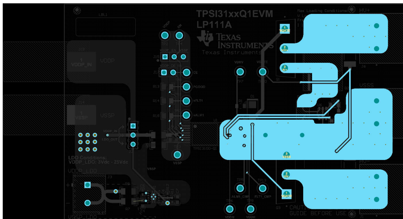
图 9-7. 信号层 2
