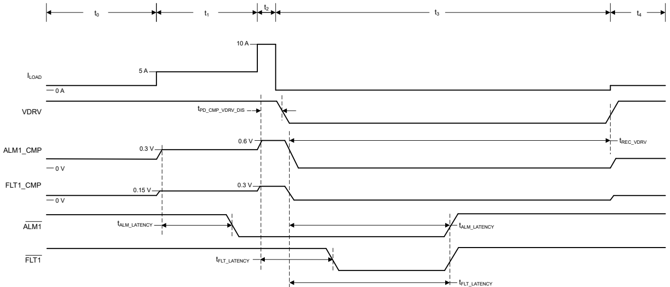
图 9-2. 过流保护的典型时序和行为
