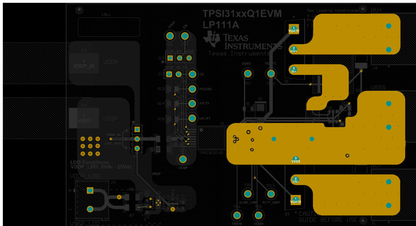
图 9-6. 信号层 1
