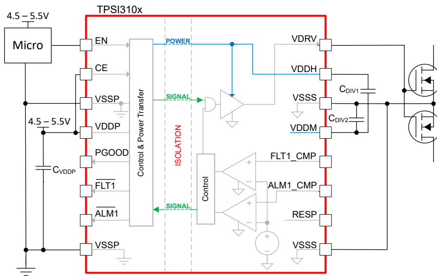
图 8-9. 简化版原理图
