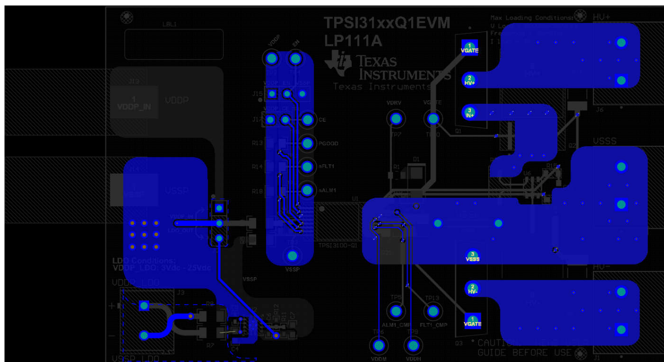
图 9-5. 底层
