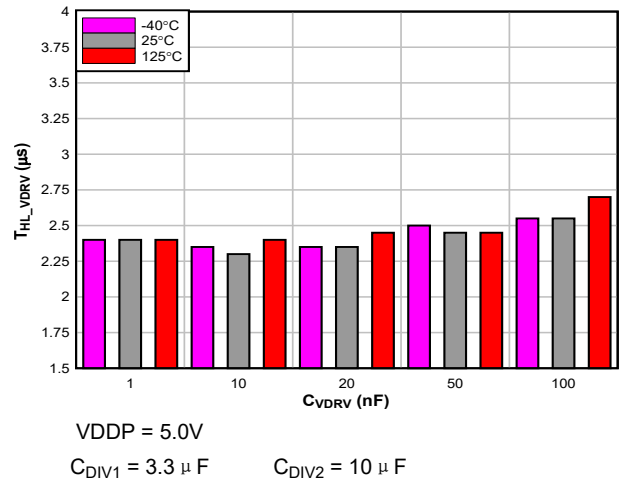
图 6-6. t_{HL\_VDRV} 与 C_{VDRV}
