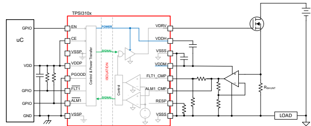
TPSI3100 简化原理图
