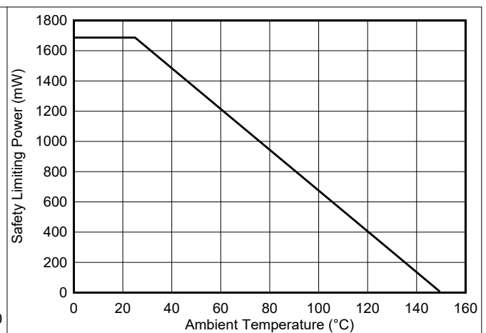
图 5-3. 安全相关限制功率的热降额曲线 (根据 VDE 标准)
