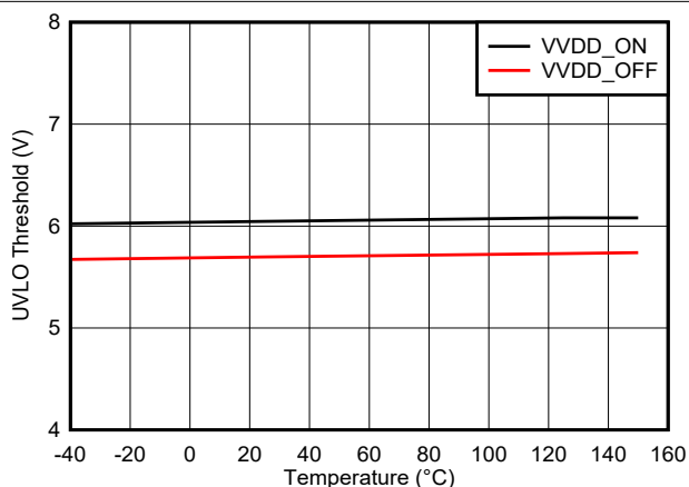
图 5-17. VDD 5V UVLO 阈值与温度间的关系
