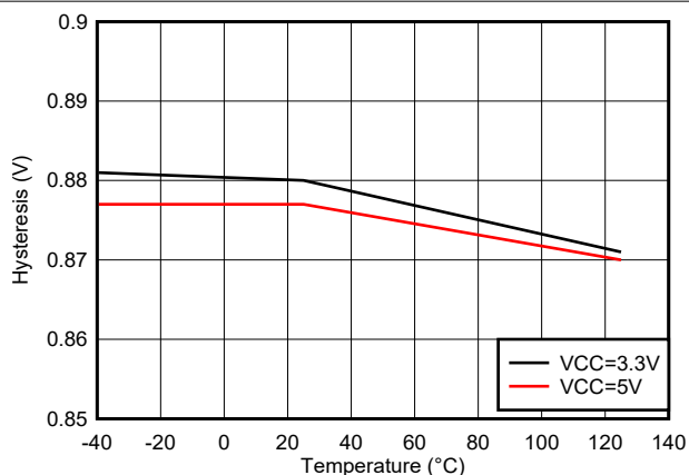
图 5-21. IN/EN 迟滞与温度间的关系
