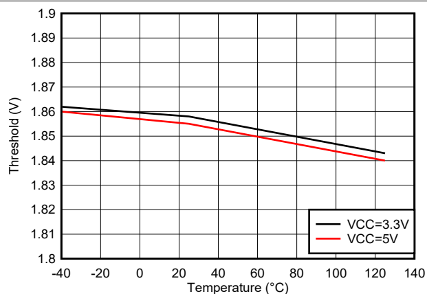
图 5-23. IN/EN 高阈值
