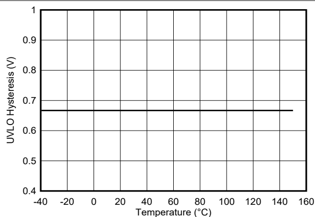
图 5-20. VDD 8V UVLO 迟滞与温度间的关系
