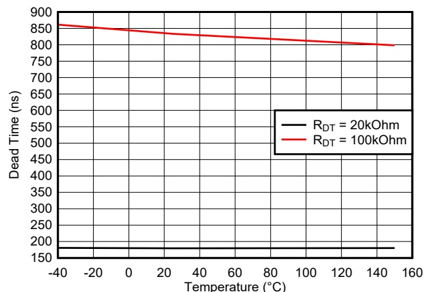
图 5-24. 死区时间与温度之间的关系 ( R_{DT} = 20k\Omega 和 100k\Omega )
