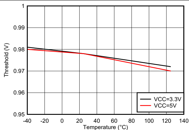
图 5-22. IN/EN 低阈值
