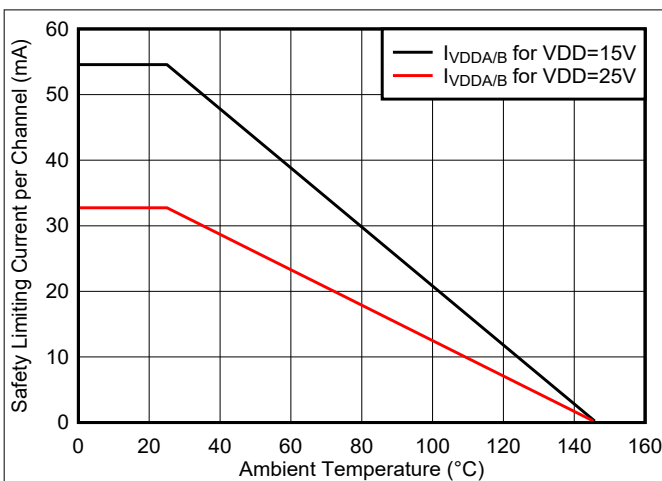
图 5-2. 根据 VDE 标准限制电流的热降额曲线 (两个通道同时运行时每个通道的电流)
