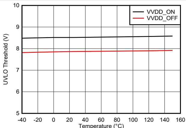
图 5-19. VDD 8V UVLO 阈值与温度间的关系
