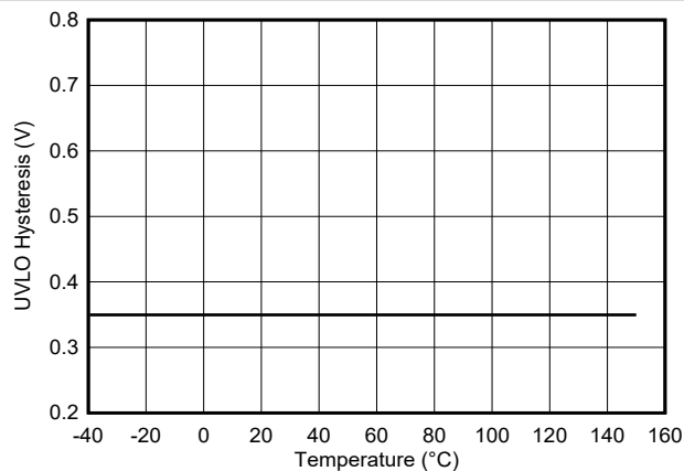
图 5-18. VDD 5V UVLO 迟滞与温度间的关系
