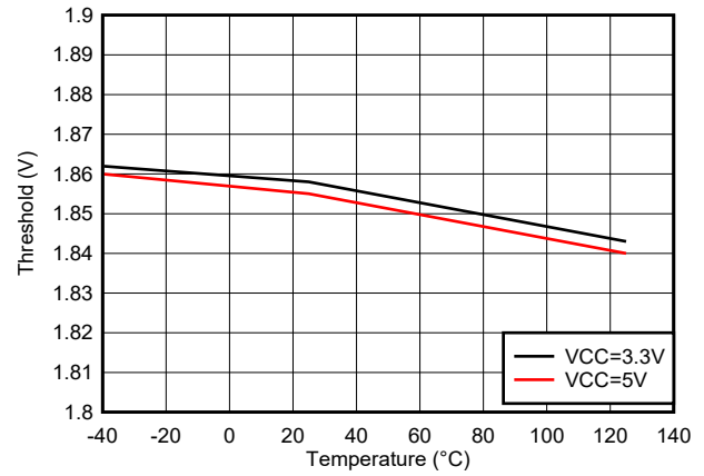
图 5-23. IN/EN 高阈值
