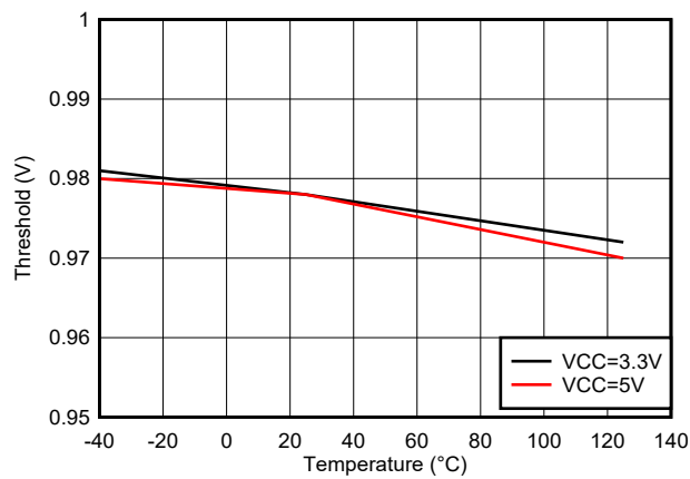
图 5-20. IN/EN 低阈值
