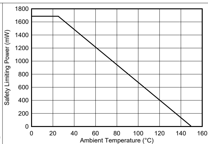
图 5-2. 安全相关限制功率的热降额曲线 (根据 VDE 标准)
