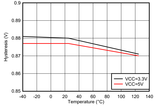
图 5-19. IN/EN 迟滞与温度之间的关系
