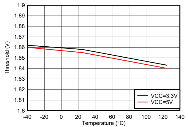
图 5-21. IN/EN 高阈值
