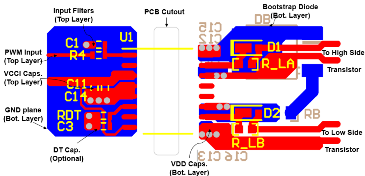
图 10-1. 布局示例
