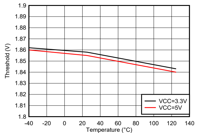
图 5-21. IN/EN 高阈值
