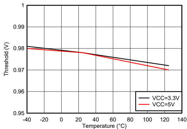
图 5-20. IN/EN 低阈值
