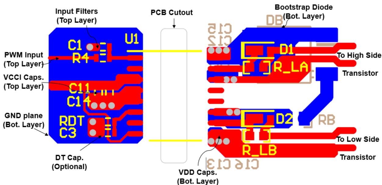
图 10-1. 布局示例
