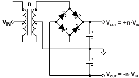
图 9-7. 具有中心抽头次级的桥式整流器可实现双极输出
