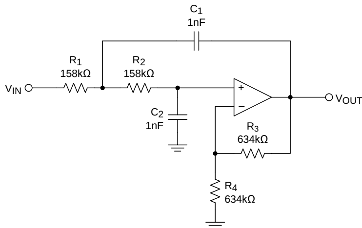
图 30. 1kHz Sallen-Key 低通滤波器及相应值
