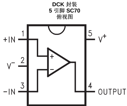
引脚功能: LMV551-Q1
