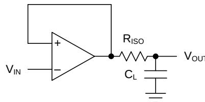
图 28. 隔离电阻器补偿
