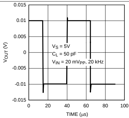
图 7. 小信号瞬态响应
