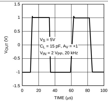
图 8. 大信号瞬态响应
