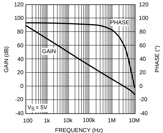
开环增益和相位与频率间的关系
