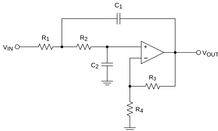
图 29. 两极 Sallen-Key 低通滤波器
