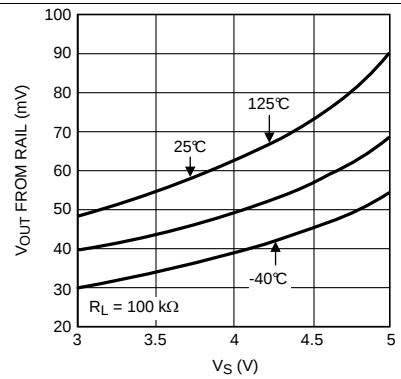
图 22. 正输出摆幅与电源电压间的关系
