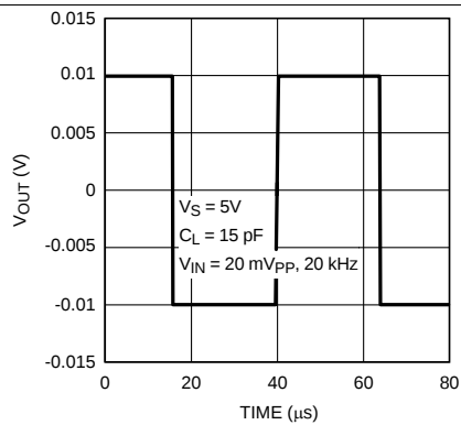
图 7. 小信号瞬态响应
