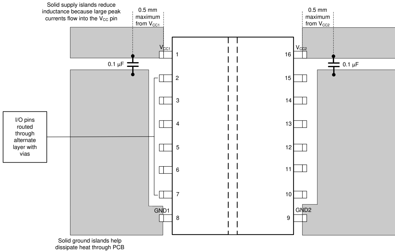
图 11-1. Layout Example
