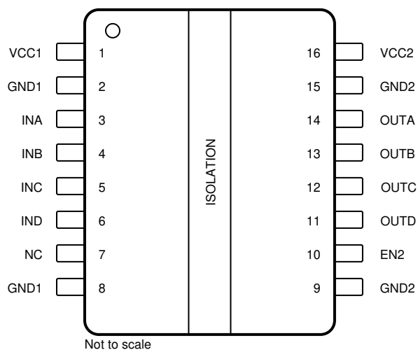
图 6-1. ISO6740-Q1 DW 封装 16 引脚 SOIC-WB 顶视图
