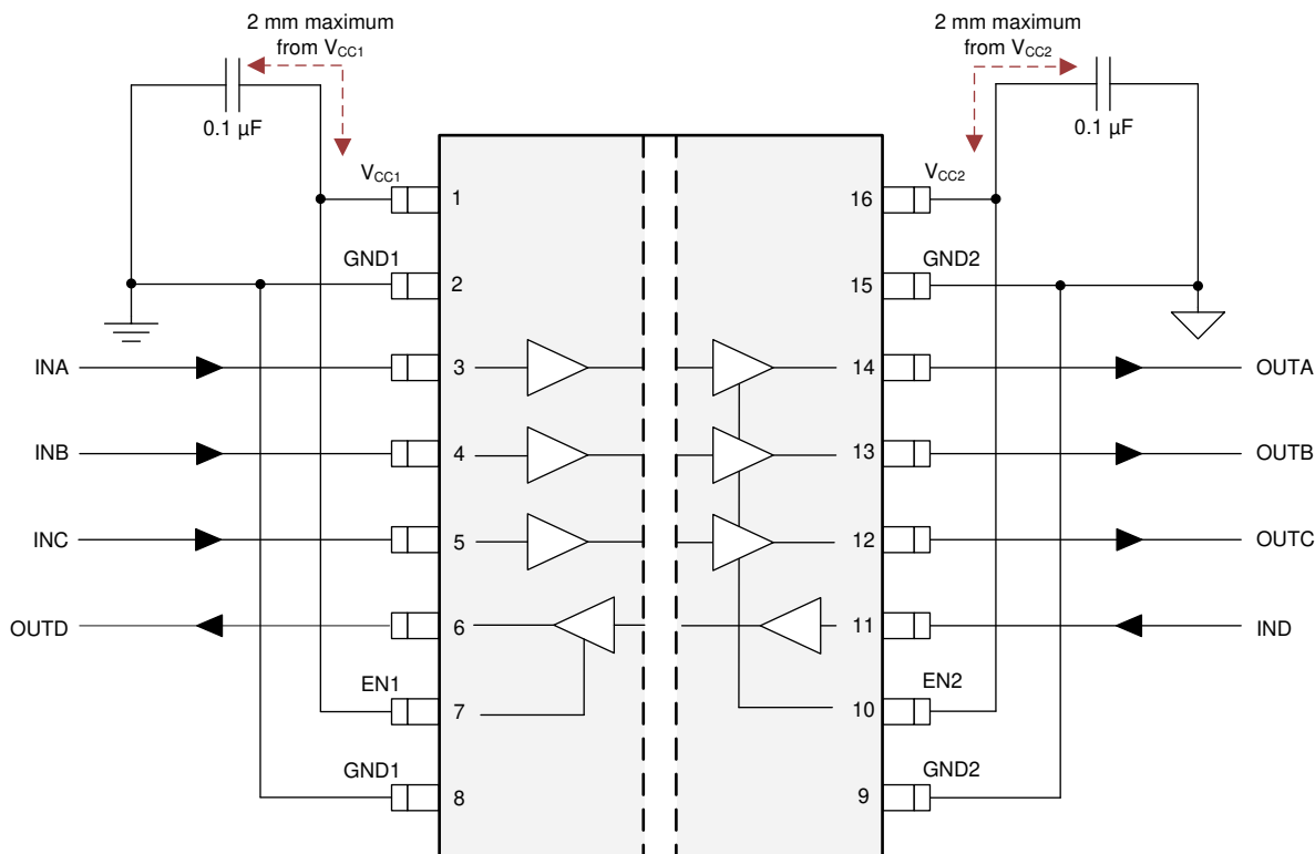
图 10-2. 典型 ISO674x-Q1 电路连接
