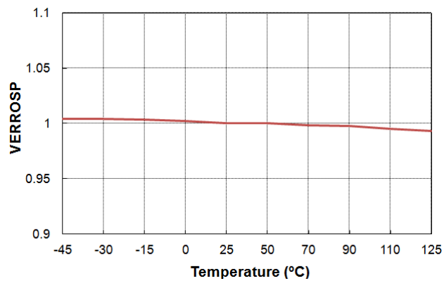
图 39. VERROSP 与温度的关系
