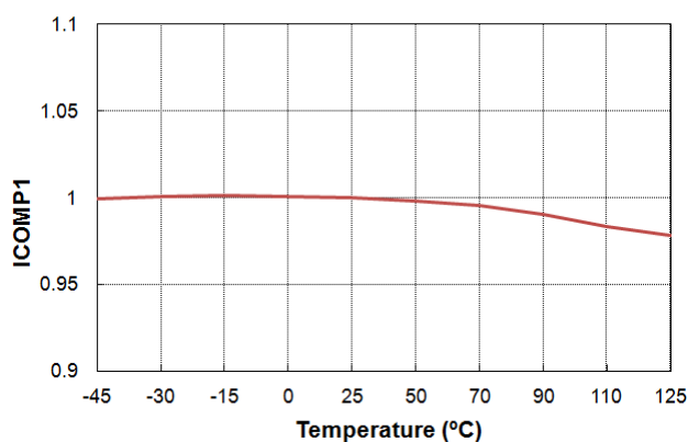
图 21. ICOMP1 与温度的关系
