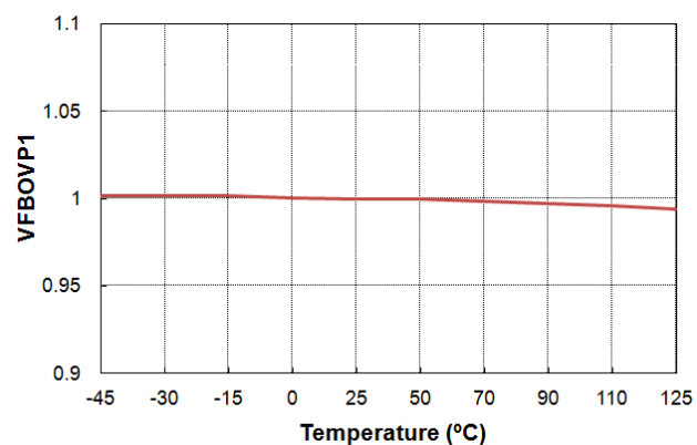
图 37. VFBOVP1 与温度的关系
