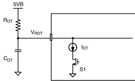
图 72. RDT 引脚的内部电流源
