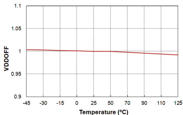
图 18. VDDOFF 与温度的关系
