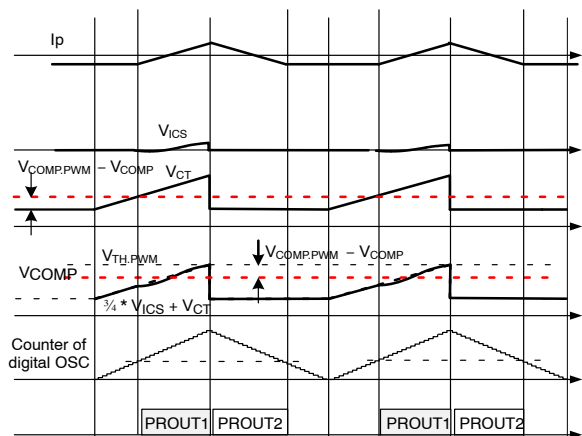
图 60. PWM 运行的主要波形
