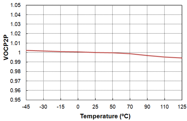
图 50. VOCP2P 与温度的关
