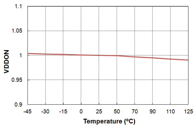
图 17. VDDON 与温度的关系
