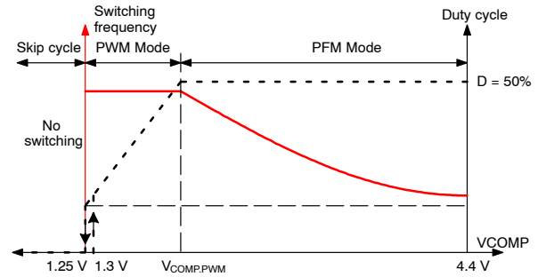
图 58. 随 COMP 电压变化的模式
