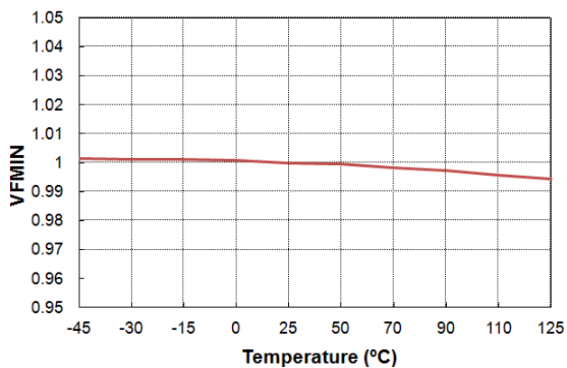
图 6. VFMIN 与温度的关系
