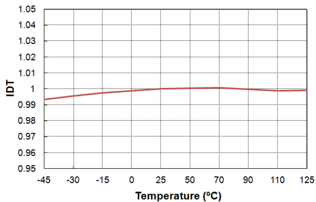
图 5. IDT 与温度的关系
