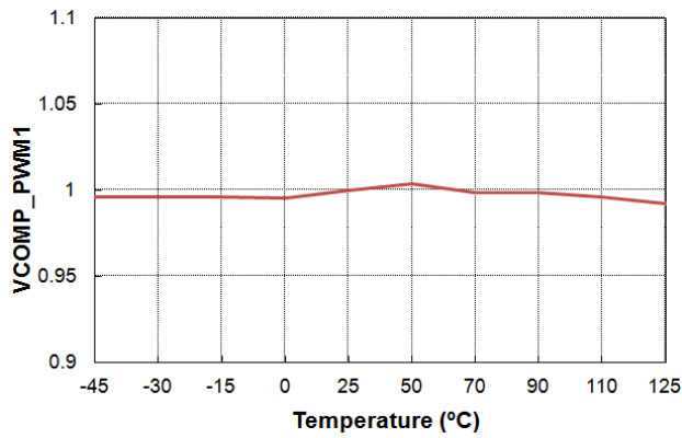
图 24. VCOMP_PWM 与温度的关系
