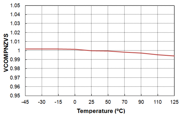
图 53. VCOMPNZVS 与温度的关系
