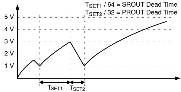
图 73. RDT 引脚的多功能操作
