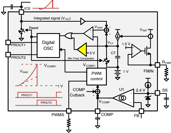
图 74. 最小开关频率设置
