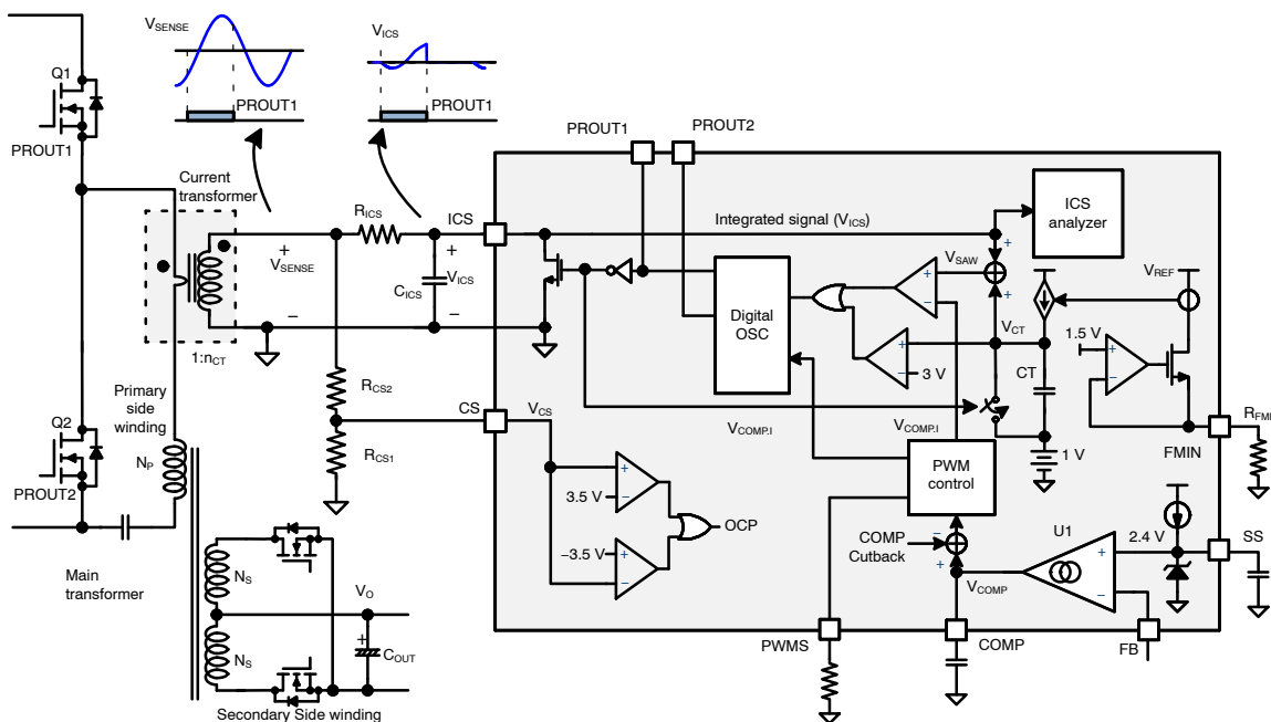
图 83. 用于电流感测和软启动的基本应用电路
