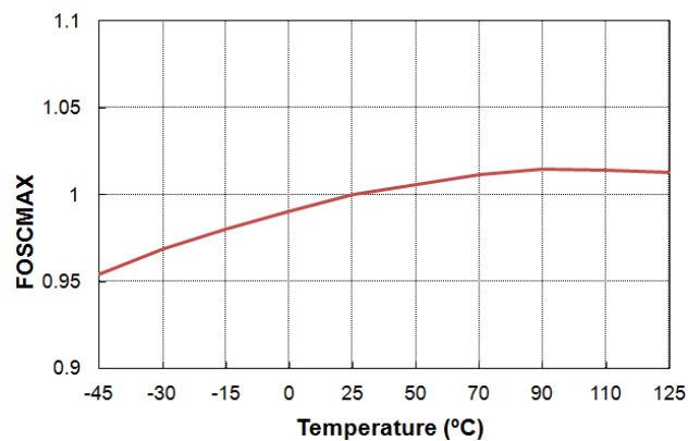
图 9. FOSCMAX 与温度的关系
