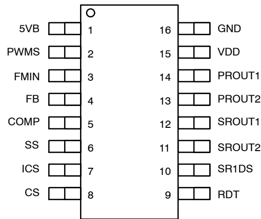
图 1. 引脚分配
