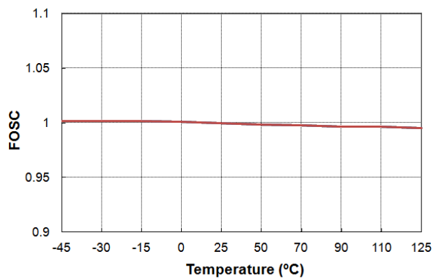
图 8. FOCS 与温度的关系
