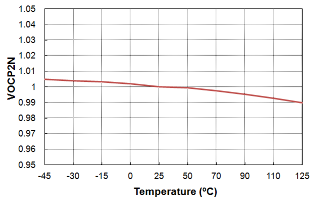
图 51. VOCP2N 与温度的关系
