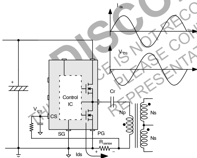
图 24. 全波检测
