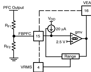
图 25. 二级 PFC 方案
