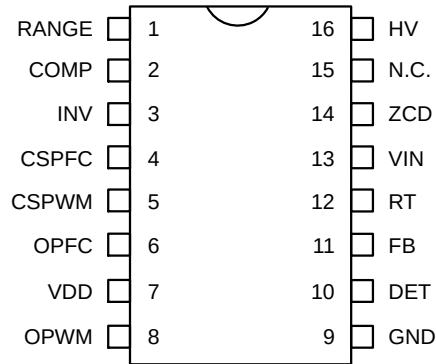
图 3. 引脚布局
