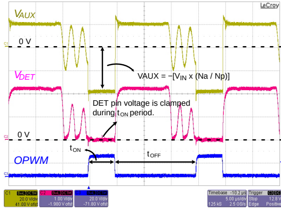
图 42. V_{AUX} 和 V_{IN} 之间的关系
