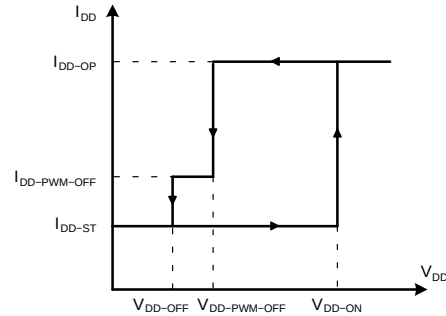
图 37. V_{DD} 与 I_{DD-OP} 特性曲线
