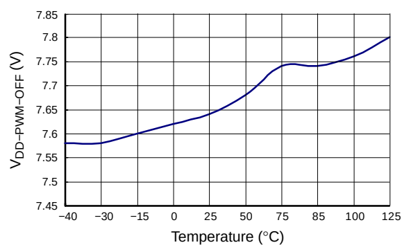
图 5. PWM 关断阈值电压
