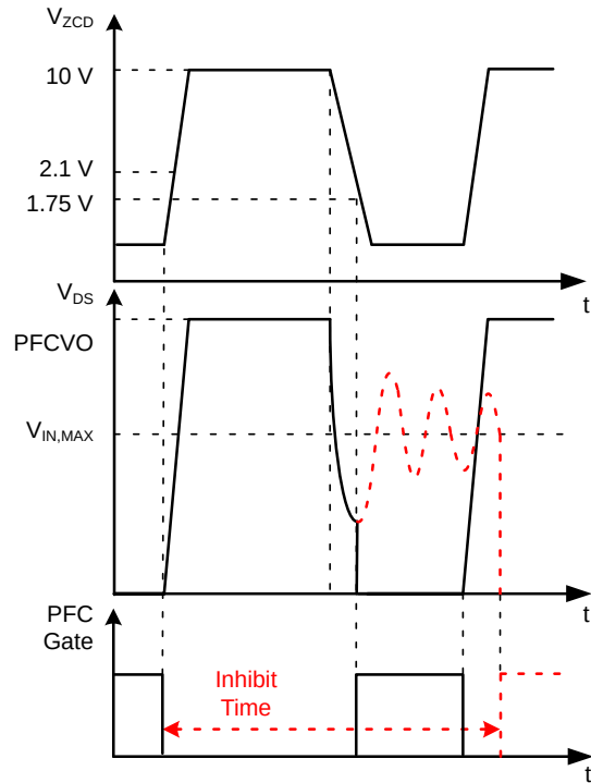
图 30. PFC 零电流检测的工作波形
