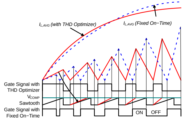
图 26. 使用和不使用 THD 优化器情况下固定导通时间的工作波形
