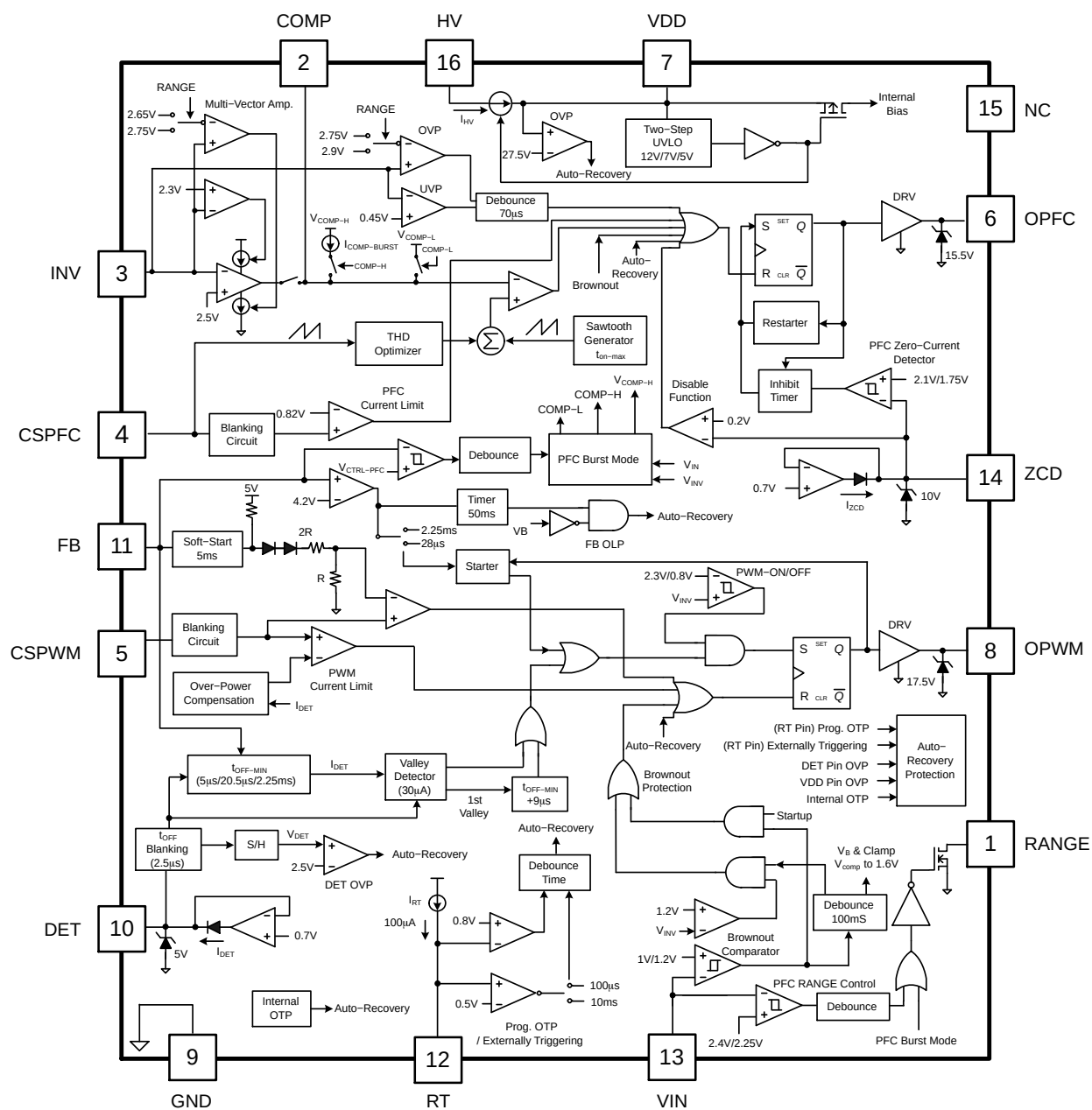
图 2. 功能框图
