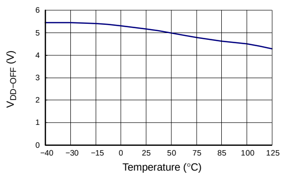
图 6. 关断阈值电压
