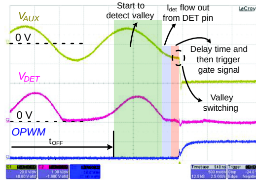
图 41. 谷底检测的测量波形
