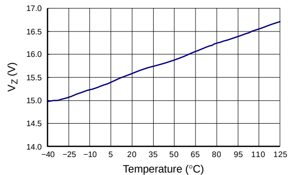
图 11. PFC 栅极输出箱位电压
