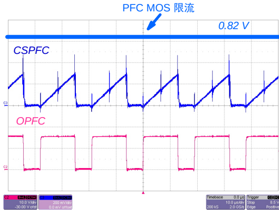
图 32. 逐周期限流
