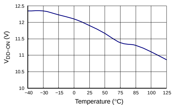
图 4. 导通阈值电压
