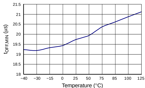
图 19. V_{FB} = V_G 的 PWM 最小关断时间
