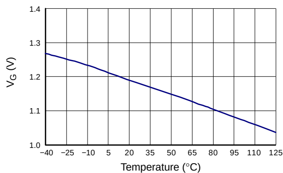
图 17. 绿色关闭模式在 V_{FB} 处开始
