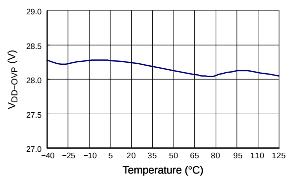
图 7. V_{DD} 过压保护阈值
