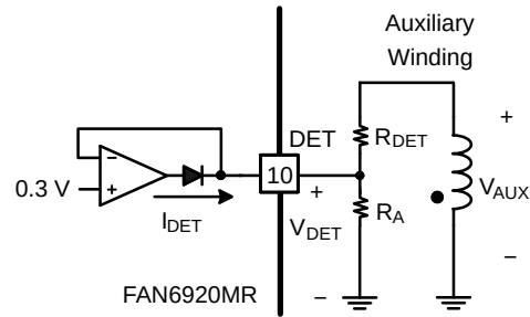
图 40. 波谷检测
