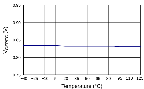
图 13. PFC 峰值限流电压
