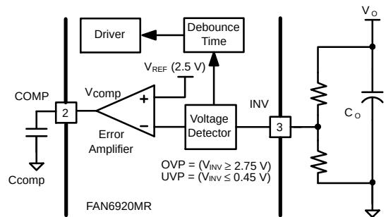
图 31. 零电流检测的内部模块
