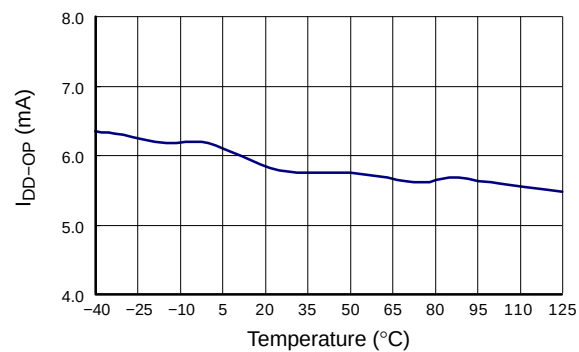
图 9. 工作电流
