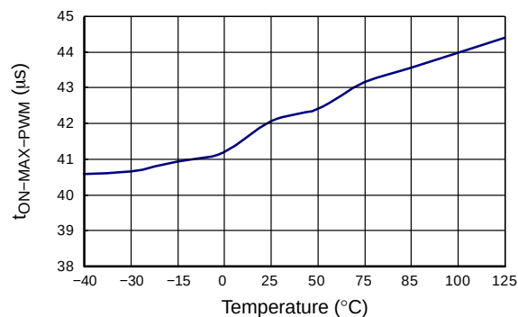
图 15. PWM 最大导通时间
