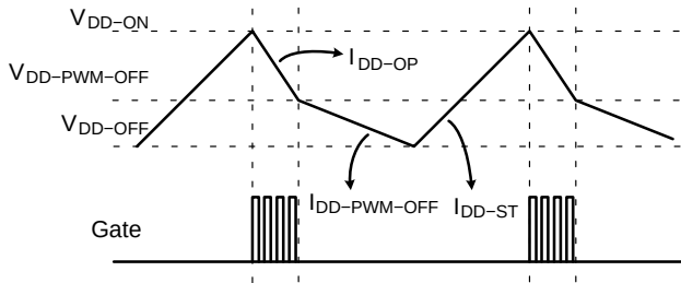
图 38. 打嗝模式操作时 V_{DD} 电压和栅极信号的典型波形
