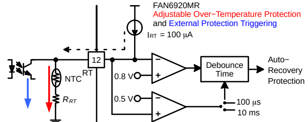
图 44. 可调过温保护
