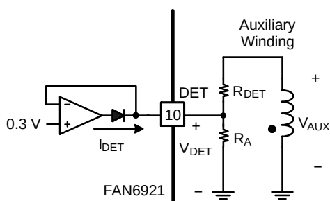
图 38. 波谷检测
