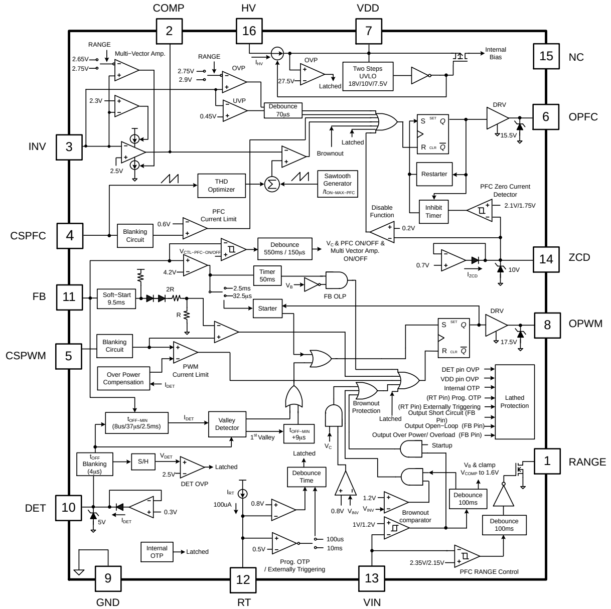
图 2. 功能框图
