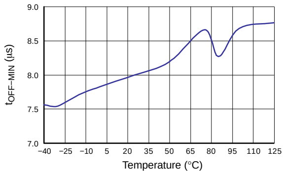
图 18. V_{FB} > V_N 的 PWM 最小关断时间
