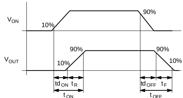
图 24. 时序图
