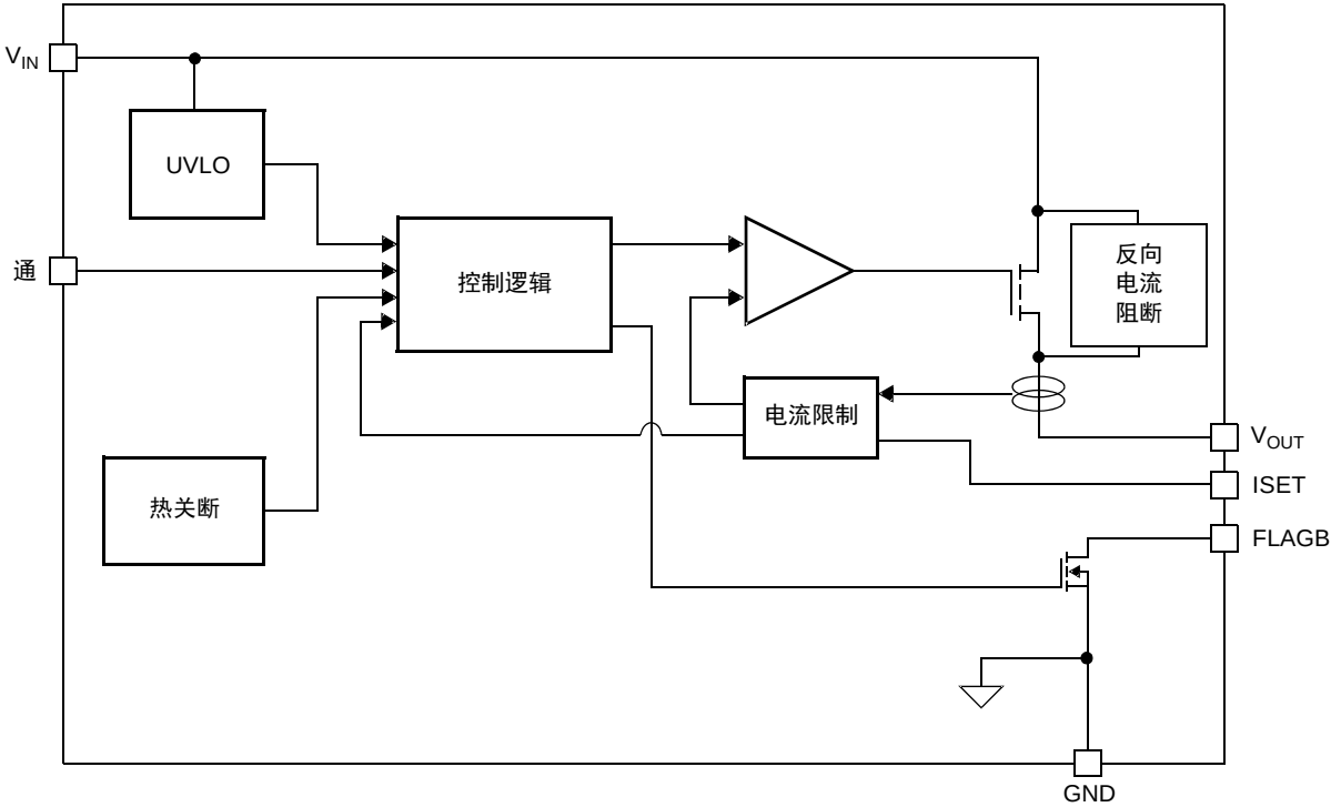
图 2. 功能框图
