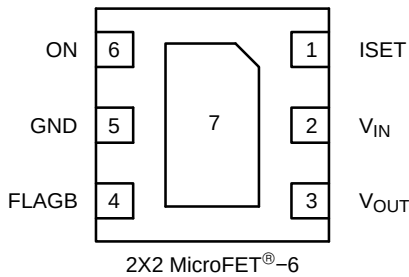
图 3. 引脚布局
