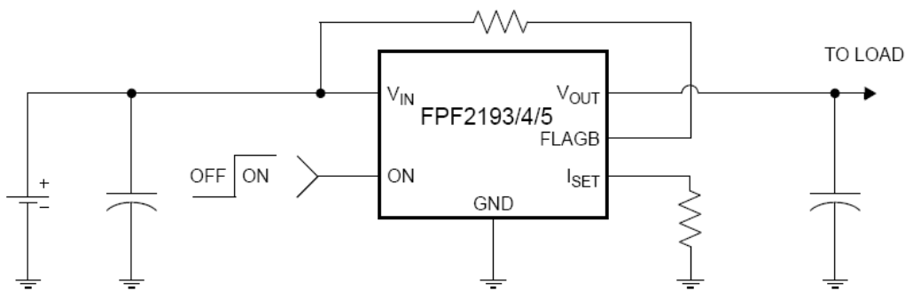
图1. 典型应用
