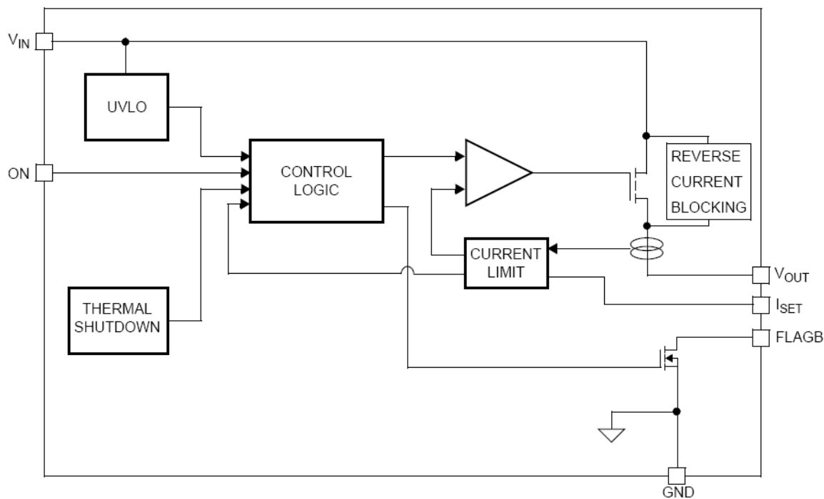
图2. 功能框图
