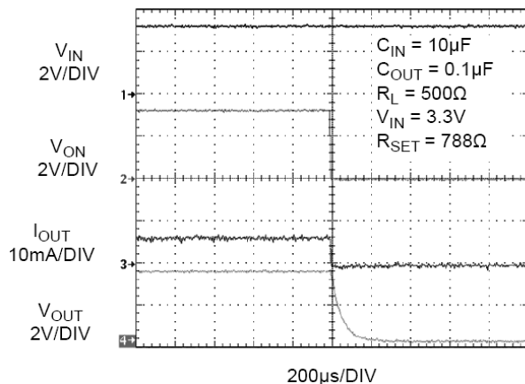
图19. t_{OFF} 响应
