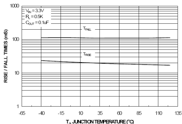
图15. t_{RISE} / t_{FALL} 与 温度的关系
