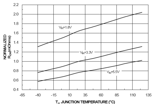
图13. R_{ON} 与温度的关系
