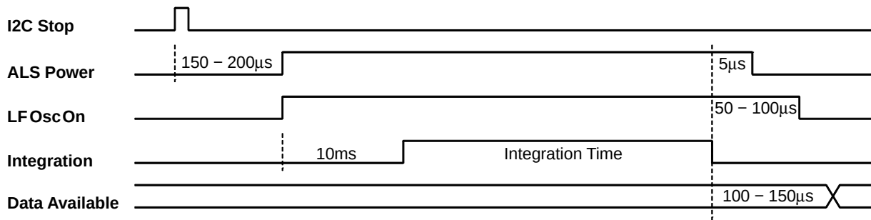
Figure 27. ALS One-Shot Timing
