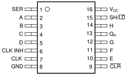
图 4-2. D 或 PW 封装，16 引脚 SOIC 或 TSSOP（顶视图）
