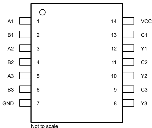
图 4-1. SN74LVC3G58 PW 封装，14 引脚 TSSOP (顶视图)
