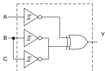
2 - Input XOR Gate
