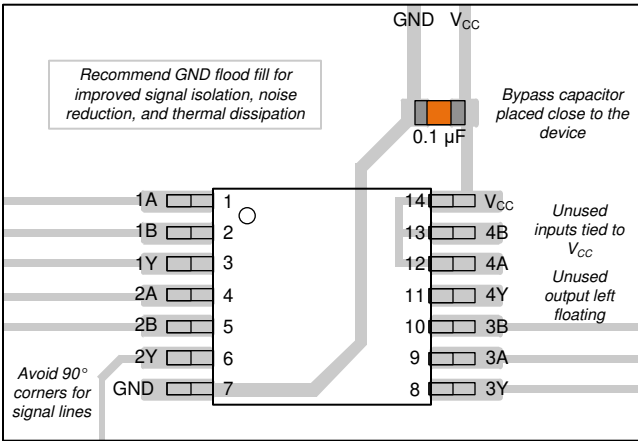
图 8-3. SN74LVC132A 的示例布局
