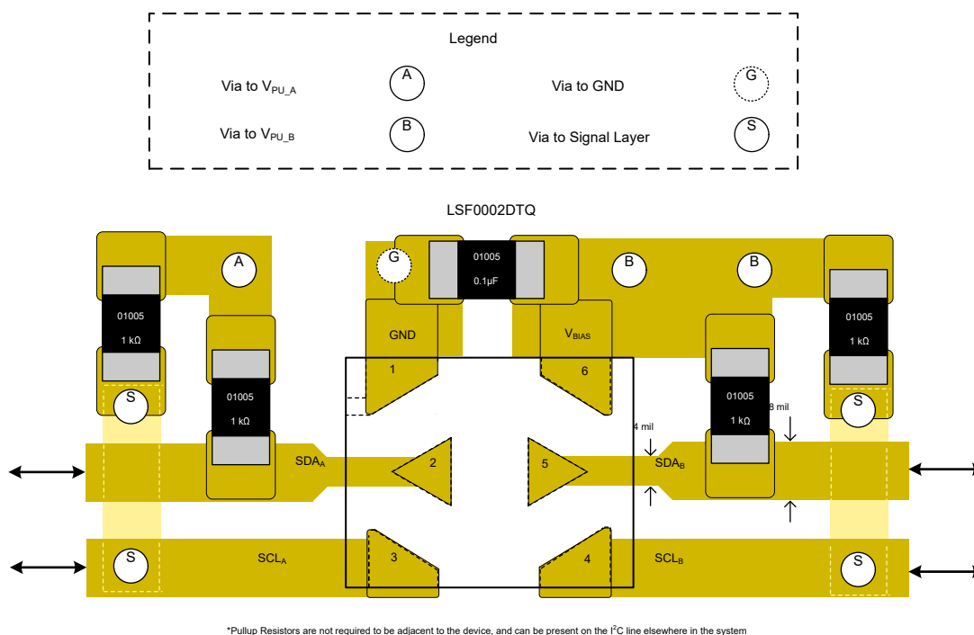
图 8-5. 短布线布局
