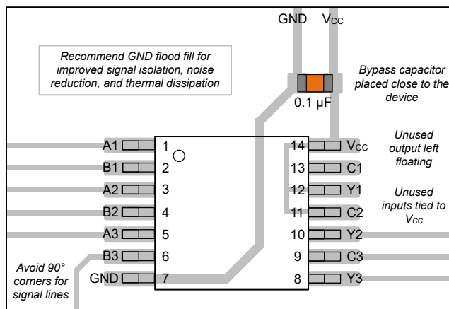
图 8-3. SN74LVC3G98 的示例布局
