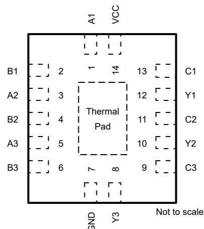
图 4-2. SN74LVC3G98 BQA 封装, 14 引脚 WQFN (顶视图)
