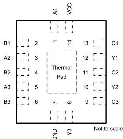
图 4-2. SN74LVC3G97 BQA 封装 , 14 引脚 WQFN ( 顶视图 )
