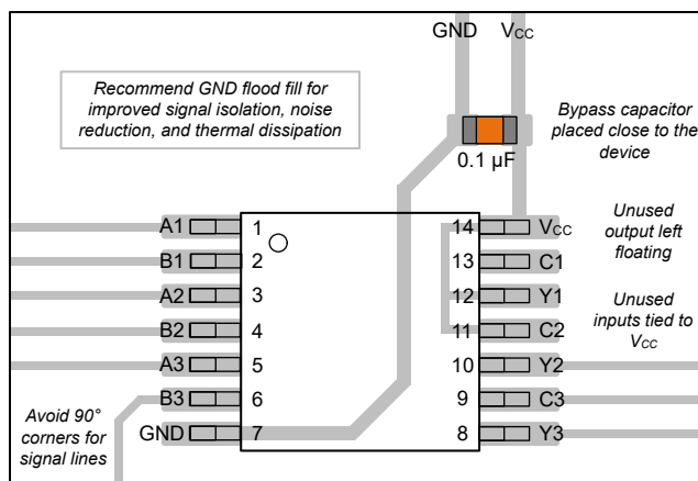
图 8-3. SN74LVC3G97 的示例布局
