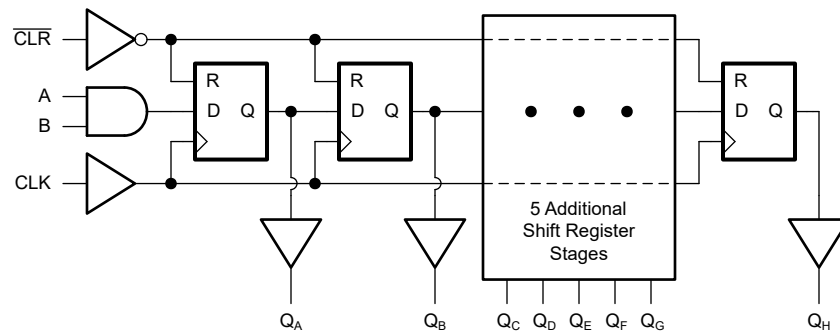
图 7-1. SN74AHC164 的逻辑图 (正逻辑)
