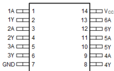
图 4-1. SN74AC16-Q1 PW 封装，14 引脚 TSSOP (俯视图)
