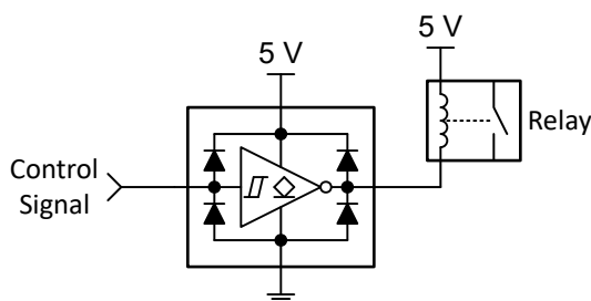
图 8-1. 典型应用框图
