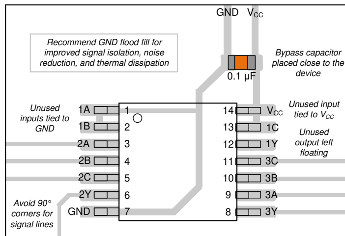
图 8-3. SN74LVC11A-Q1 示例布局
