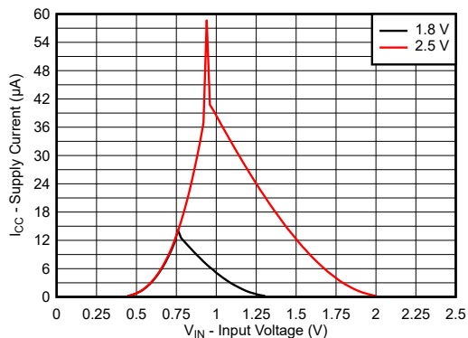
图 6-1. 输入电压范围内的电源电流, 1.8V 和 2.5V 电源
