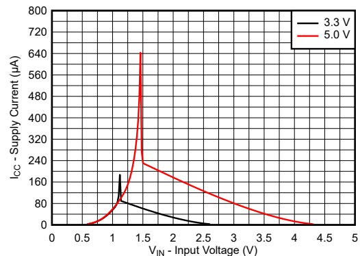
图 6-2. 输入电压范围内的电源电流, 3.3V 和 5.0V 电源
