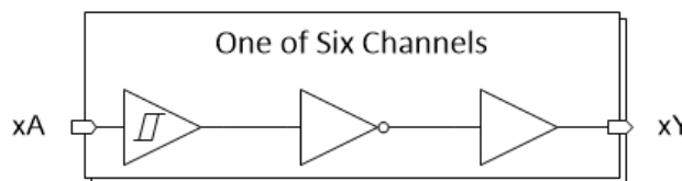
简化逻辑图
