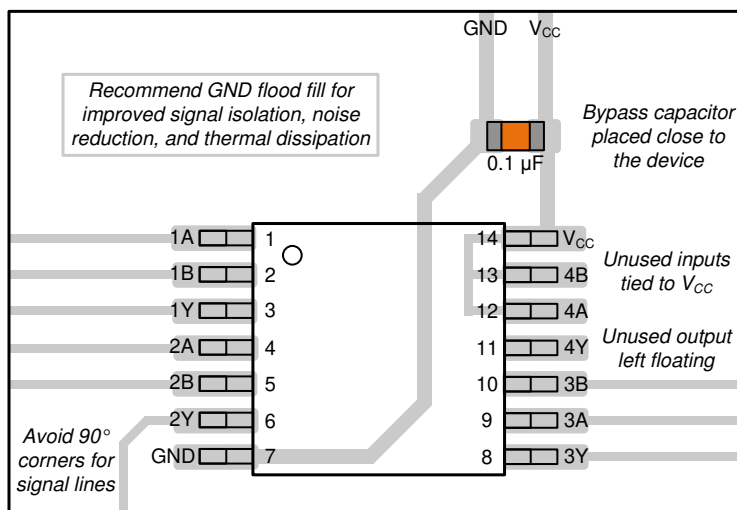
图 10-1. SN74LV6T17-EP 的示例布局
