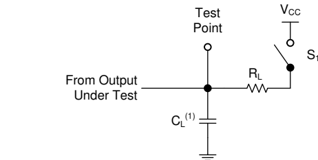
图 6-1. 开漏输出的负载电路
