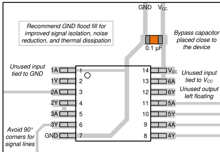
图 8-3. SN74LV6T14-EP 的示例布局
