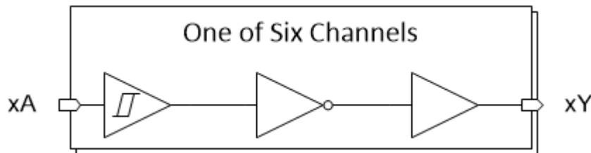
简化逻辑图 (正逻辑)
