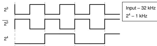
图 8-2. 应用时序图
