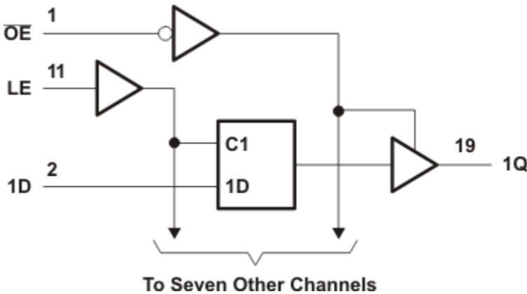
图 6-1. 逻辑图 (正逻辑)
