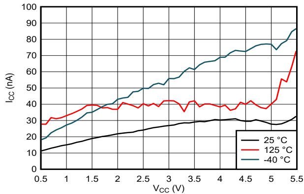
图 4-1. 电源电流与电源电压的关系
