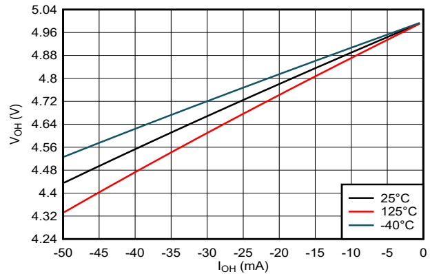
图 4-2. 高电平状态下输出电压与电流间的关系（5V 电源）
