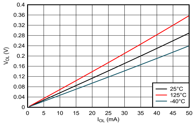
图 4-3. 低电平状态下输出电压与电流间的关系；5V 电源
