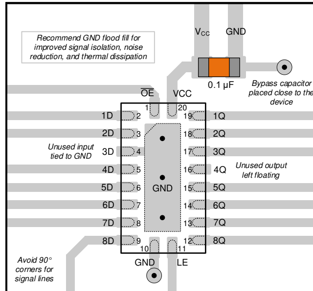
图 7-3. 采用 RKS 封装的 SN74ACT573-Q1 的示例布局
