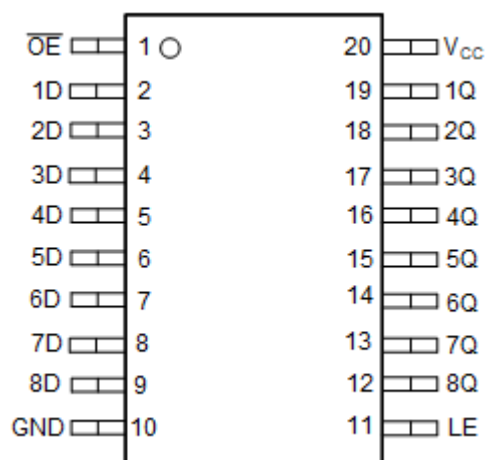
图 3-1. SN74ACT573-Q1 PW 封装，20 引脚 TSSOP (顶视图)
