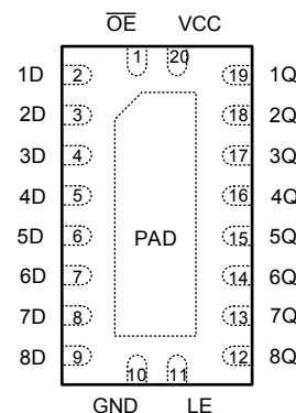
图 3-2. SN74ACT573-Q1 RKS 封装，20 引脚 VQFN (顶视图)
