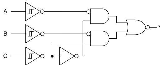
简化逻辑图
