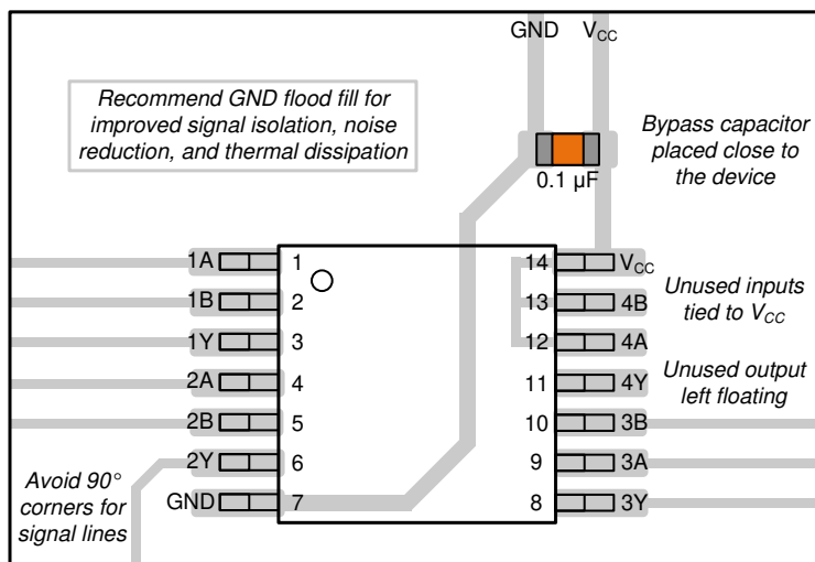
图 8-3. 示例布局 SN54SC4T86-SEP
