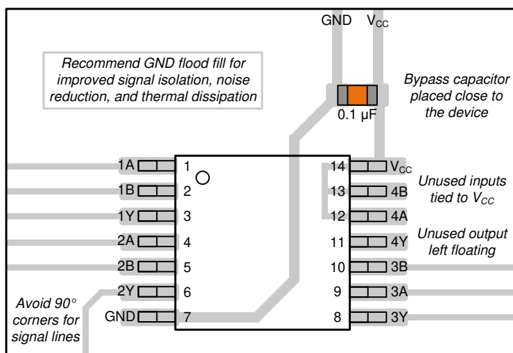
图 8-3. 示例布局 SN54SC4T32-SEP
