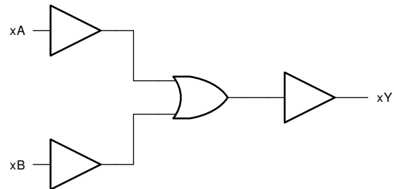
简化逻辑图
