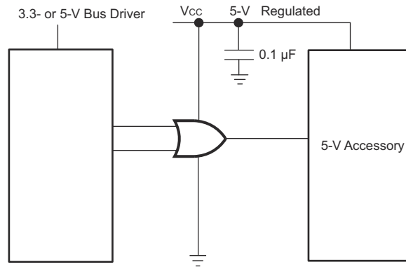
图 8-1. 单门的典型应用图
