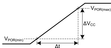
图 7-3. 已知上电状态的电源 ( V_{CC} ) 斜坡特性
