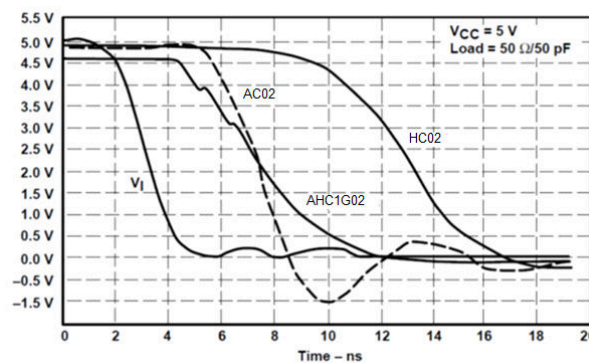
图 9-2. 应用曲线
