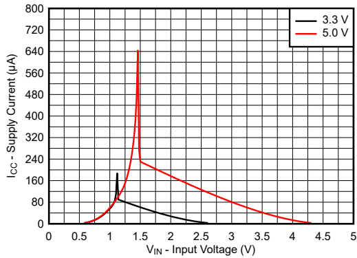
图 6-1. 3.3V 和 5.0V 输入电压电源上的电源电流
