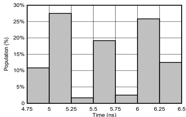
图 6-18. T_{PD} 分布；5V； T_A = -55^\circ\text{C} 至 125^\circ\text{C} (40 个样本)
