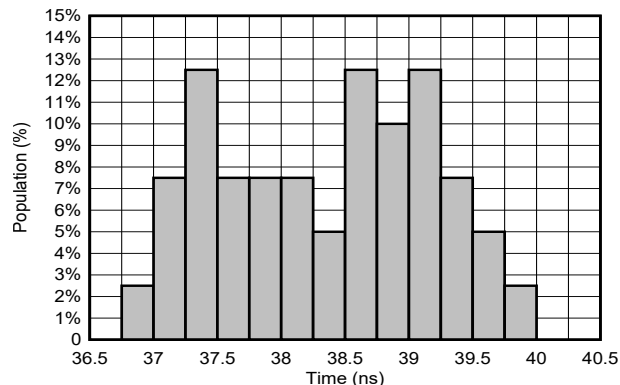
图 6-14. T_{PD} 分布；1.2V； T_A = -55^\circ\text{C} 至 125^\circ\text{C} (40 个样本)
