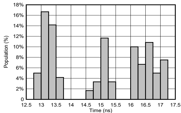
图 6-15. T_{PD} 分布；1.8V； T_A = -55^\circ\text{C} 至 125^\circ\text{C} (40 个样本)
