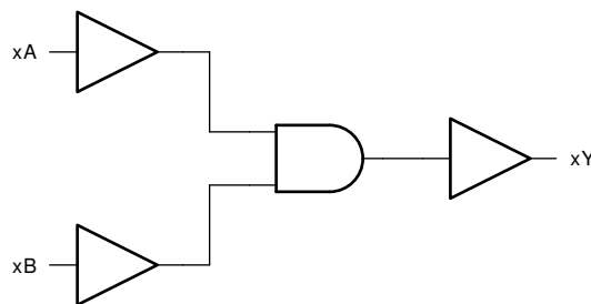
简化逻辑图
