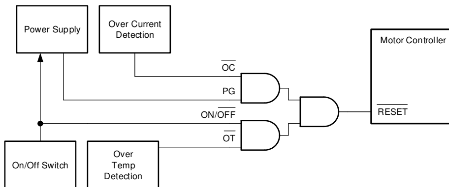
图 9-1. 典型应用框图
