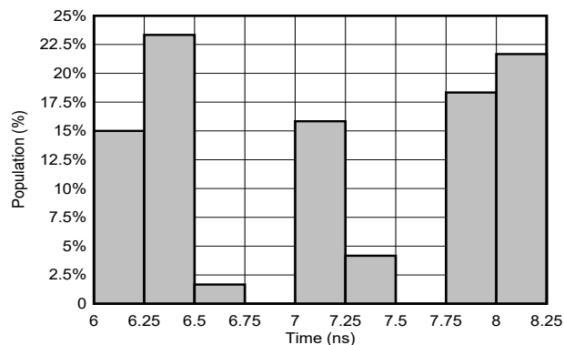
图 6-17. T_{PD} 分布；3.3V； T_A = -55^\circ\text{C} 至 125^\circ\text{C} (40 个样本)
