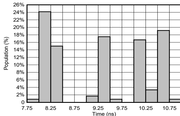
图 6-16. T_{PD} 分布；2.5V； T_A = -55^\circ\text{C} 至 125^\circ\text{C} (40 个样本)
