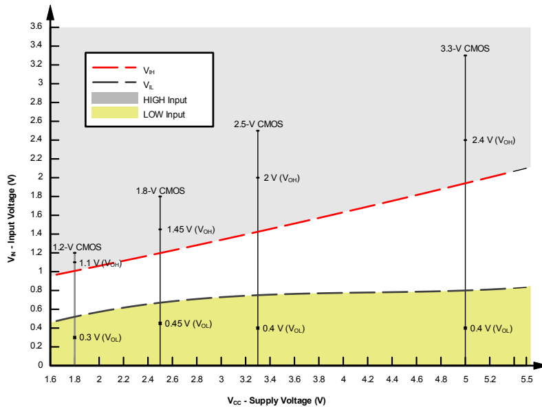
图 8-2. SCxT 输入电压电平
