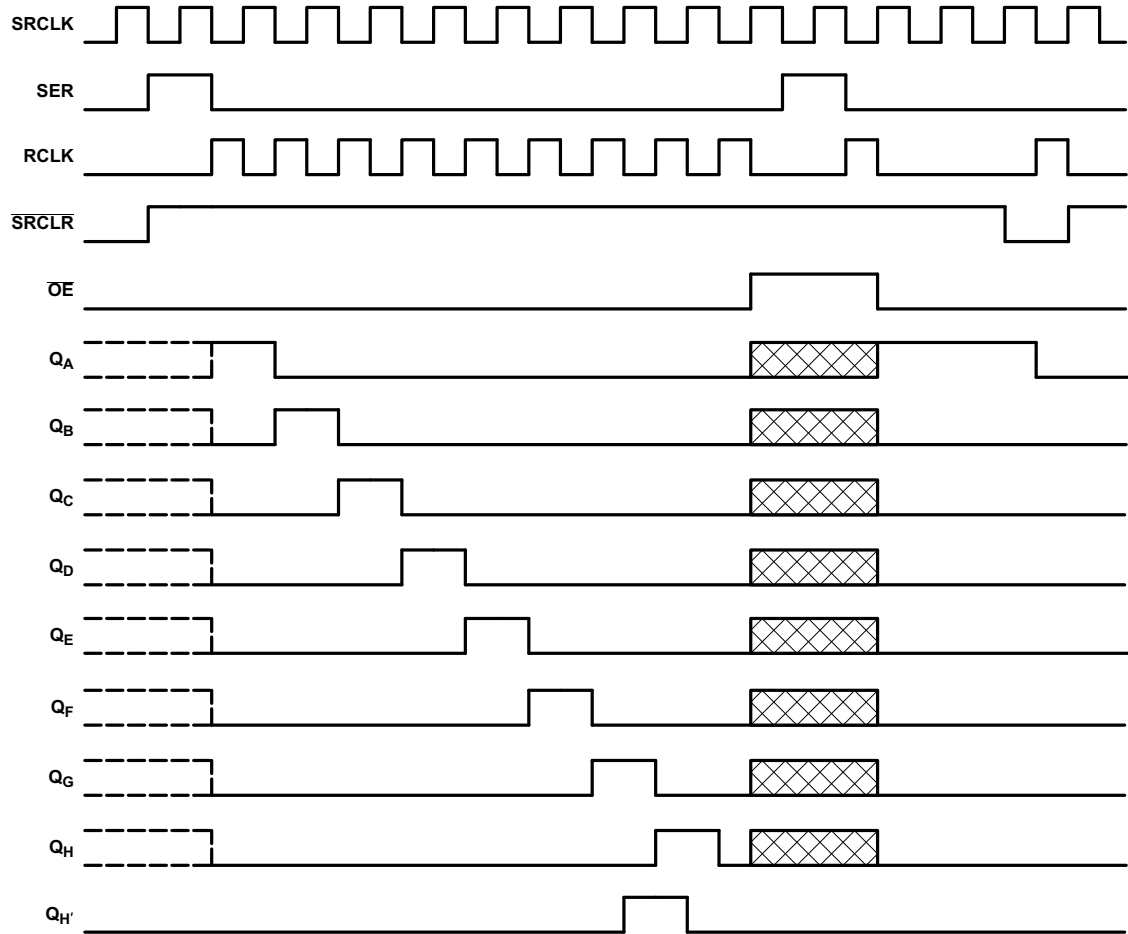
图 6-1. 时序图
