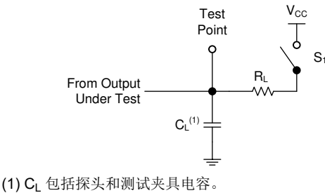
(1) C L 包括探头和测试夹具电容。 图 7-1. 开漏输出的负载电路
