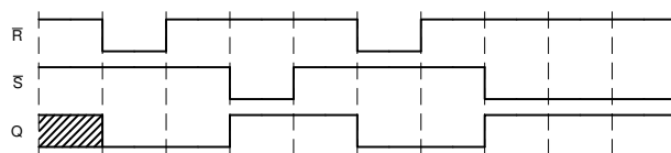
图 8-2. 应用时序图
