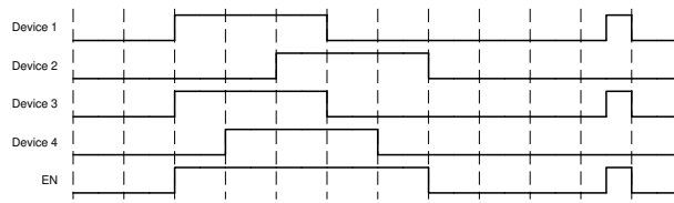
图 8-2. 应用时序图
