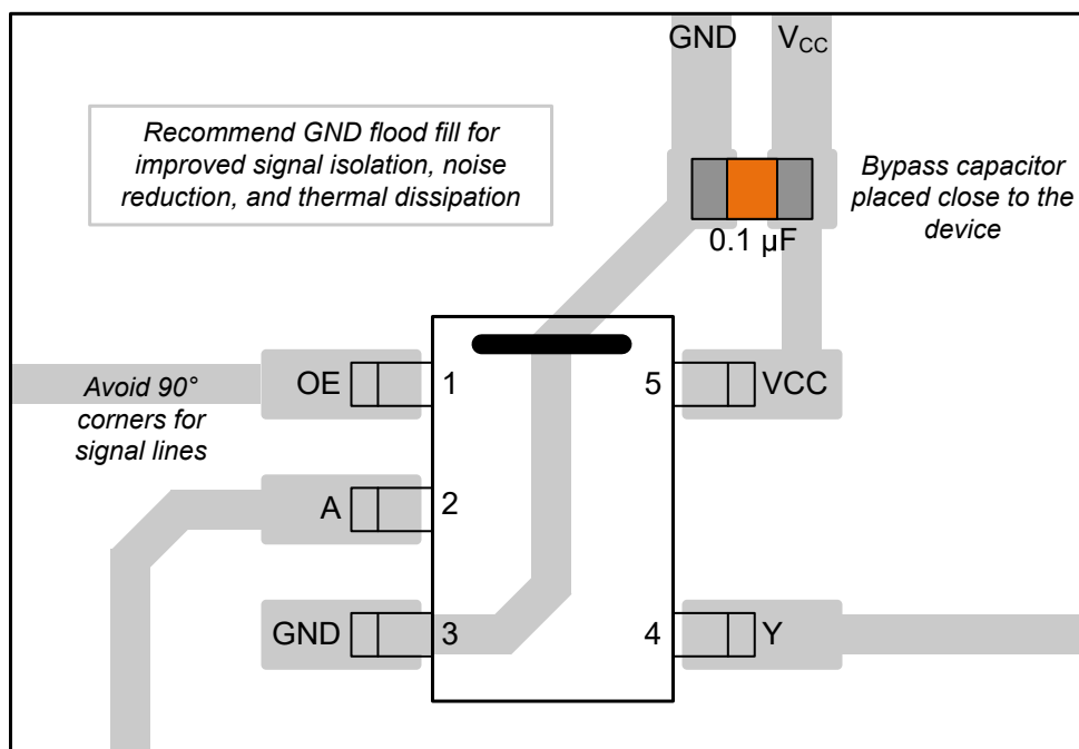
图 10-1. SN74LV1T125-Q1 的示例布局
