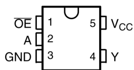
图 4-1. DCK 或 DBV 封装，5 引脚 SC70 或 SOT-23 (顶视图)
