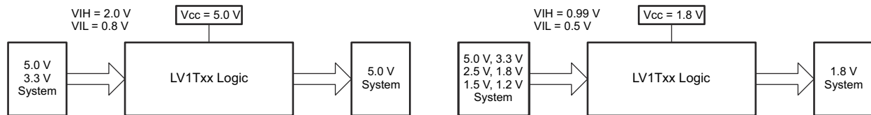
图 7-3. LVxT 升压和降压转换示例
