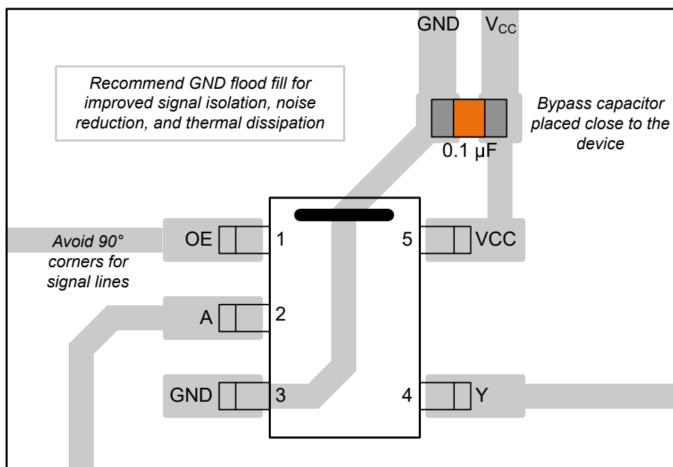
图 8-3. SN74LV1T126-Q1 的示例布局
