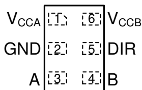
图 5-3. DRY 封装预发布，6 引脚 SON (顶视图)
