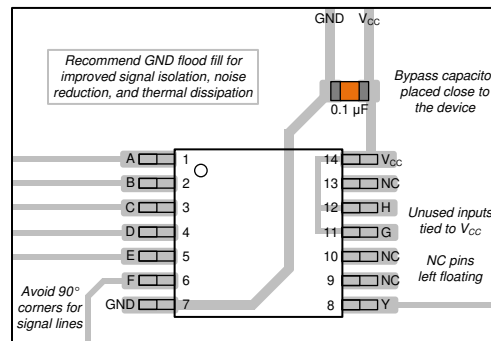
图 11. Example layout for the SN74HCS30-Q1
