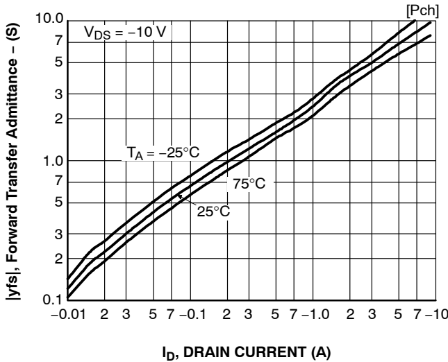
Figure 16. |y_{fs}| - I_D
